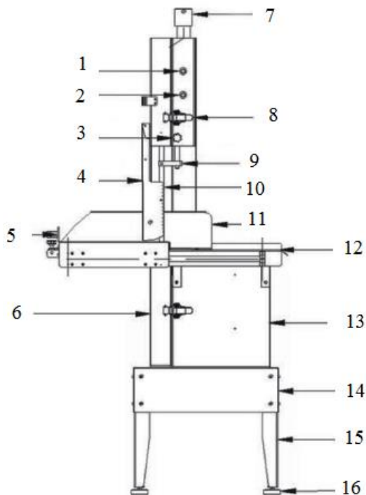
Рис. 1 Общий вид оборудования модель HR-300A. Основные детали оборудования.
