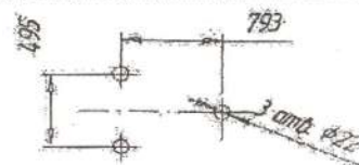
Рисунок 2. План расположения фундаментных болтов.
