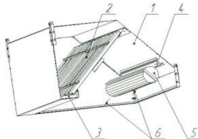
Рис.3 Схема сборки зонтов со светильниками.
