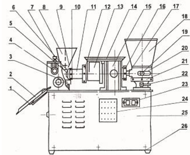
Рис1. Общий вид оборудования
