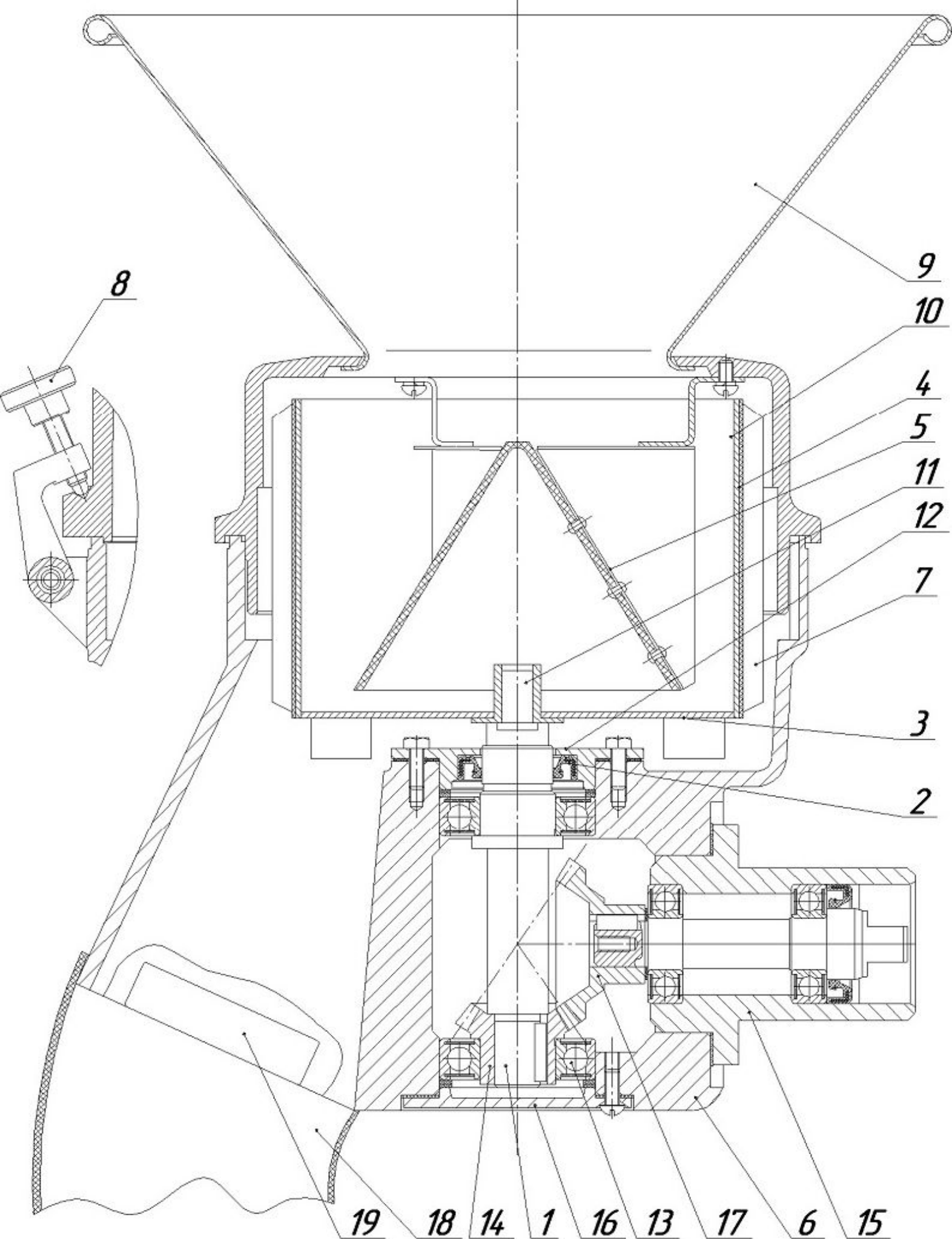
Просеиватель МП – 01
